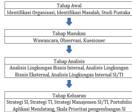
Gambar 1. Rancangan Penelitian
