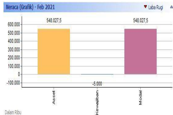
Gambar 21. Neraca (Grafik)
