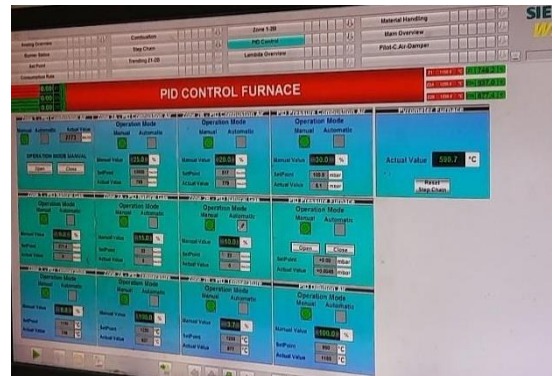
Gambar 5. Tampilan Kontrol PID
