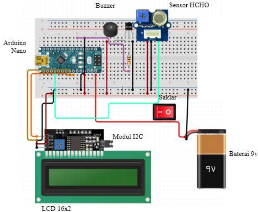
Gambar 2. Skema Rangkaian
